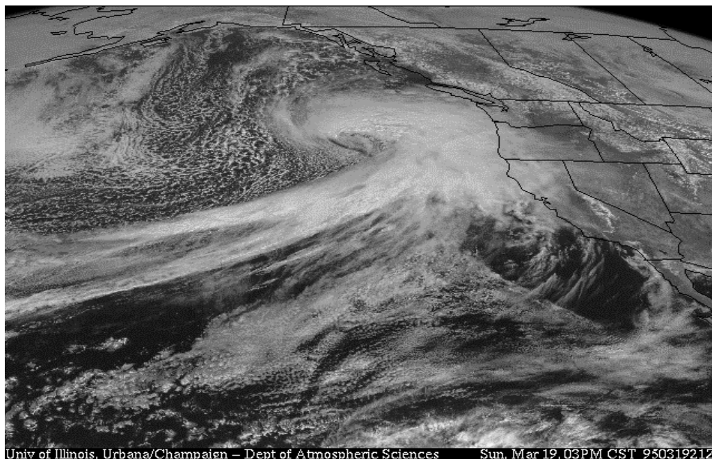
รูปที่ 38 ส่วนประกอบของ Comma Cloud
