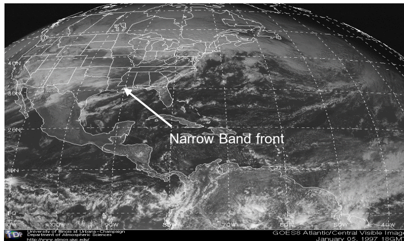
รูปที่ 31 Inactive Cold Front หรือ Narrow band
