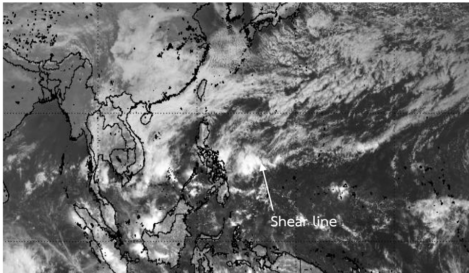
รูปที่ 46 shear line
