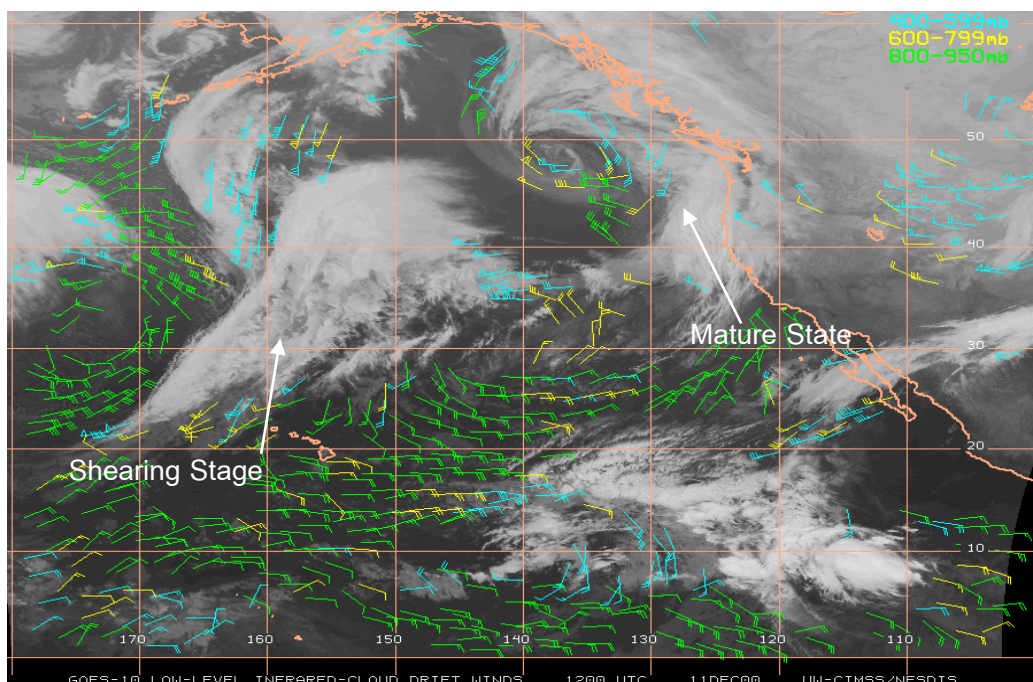
รูปที่ 41 Mature Stage and Shearing Stage
