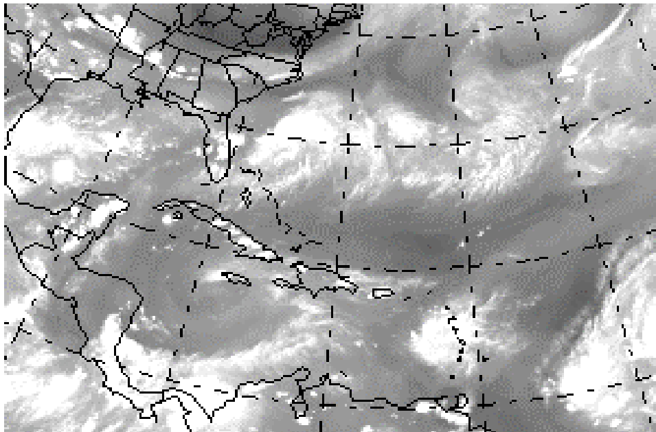
รูปที่ 48 Tropical Upper Tropospheric Trough (TUTT)
