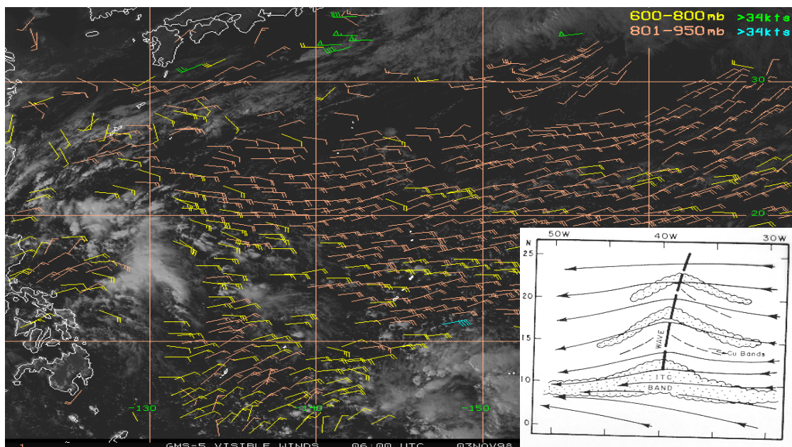
รูปที่ 47 Easterly Wave in West Pacific
