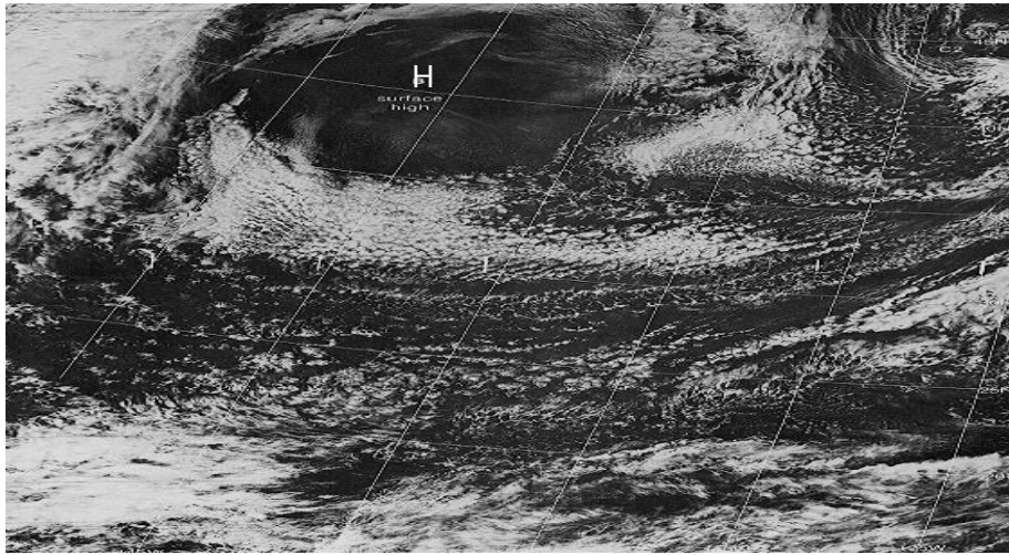
รูปที่ 29 Surface High Center
