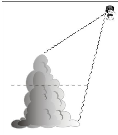
รูปที่ 15 การเกิด Contamination จากความหนาของเมฆและมุกกล้อง
