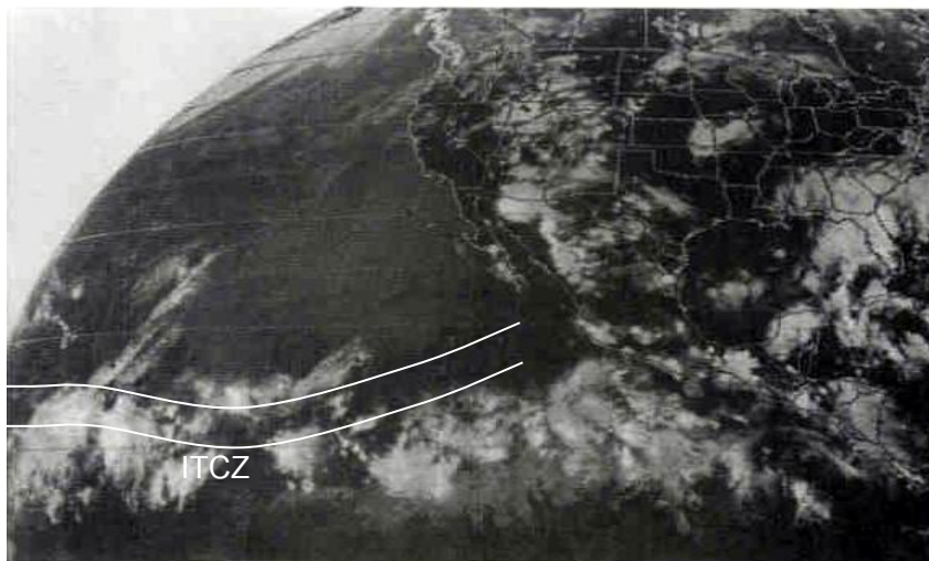
รูปที่ 49 Intertropical Convergence Zone (ITCZ)
