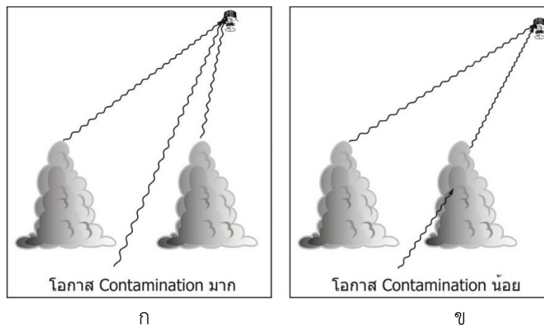
รูปที่ 16 การเกิด Contamination จากช่องว่างระหว่างเมฆ
