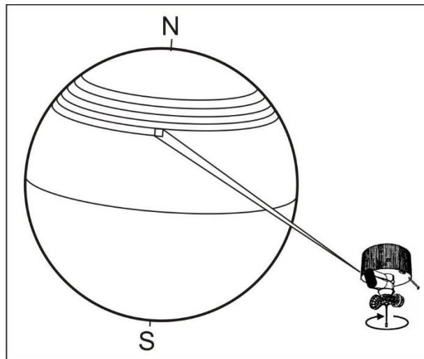
รูปที่ 2 ดาวเทียมอุตุนิยมวิทยาชนิดโคจรประจำที่
